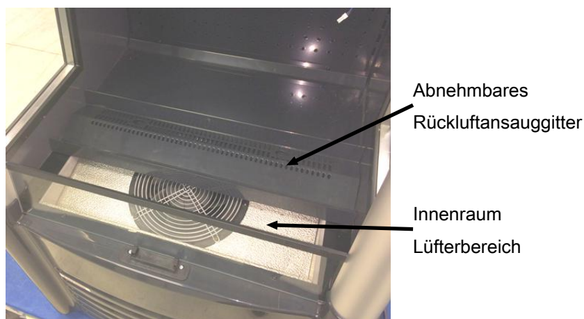
Abb. 16: abnehmbares Rückluftansaugitter
